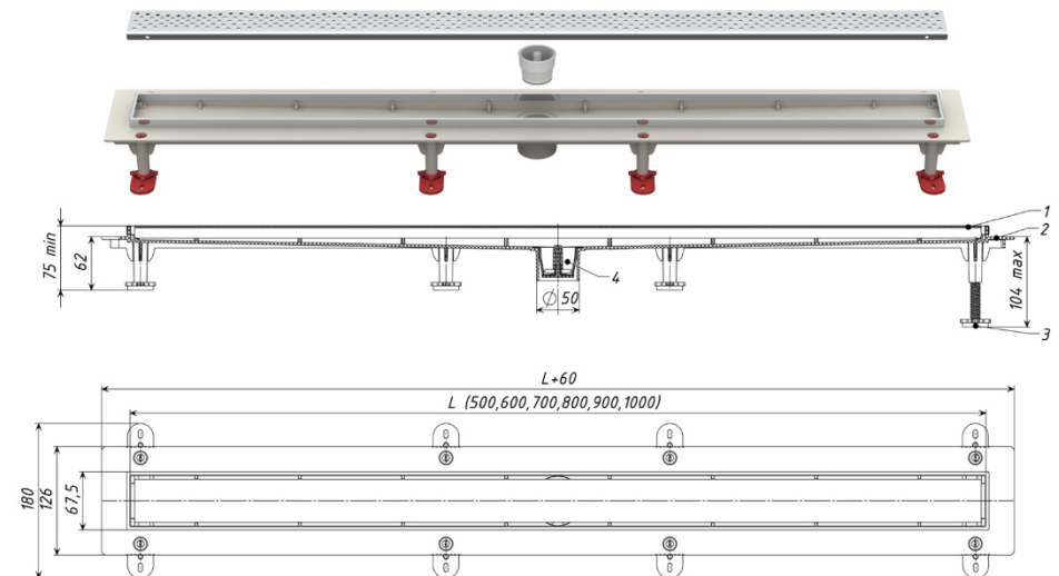
Рис. 1 – Габаритные размеры
