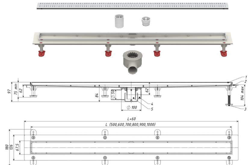
Рис. 1 – Габаритные размеры
